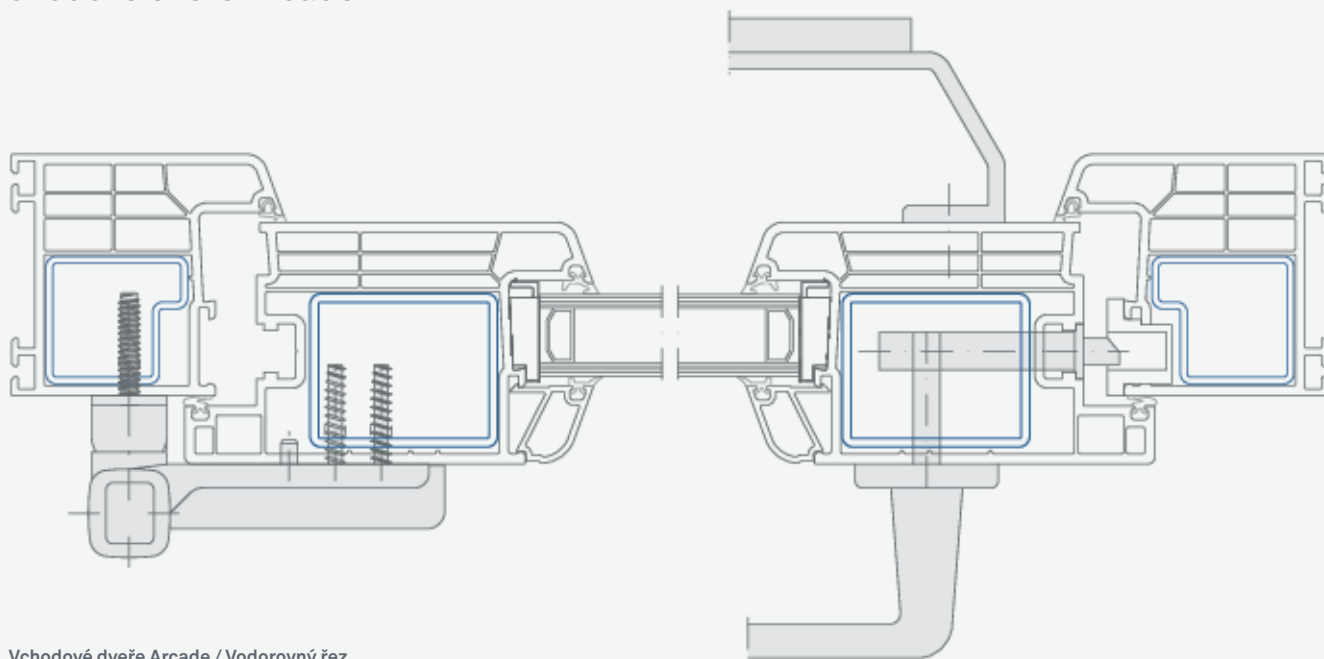
Vchodové dveře Arcade / Vodorovný řez
