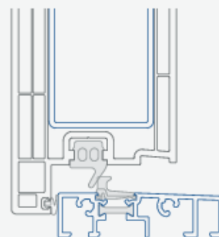
Varianta s otevíráním ven
