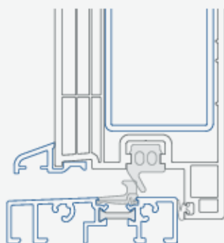
Varianta s otevíráním dovnitř
