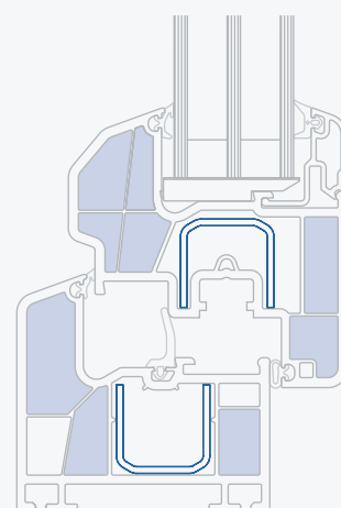
Prestige varianta s vysokou tepelnou izolací I 76.4 C4 těsnění uprostřed (MD)
