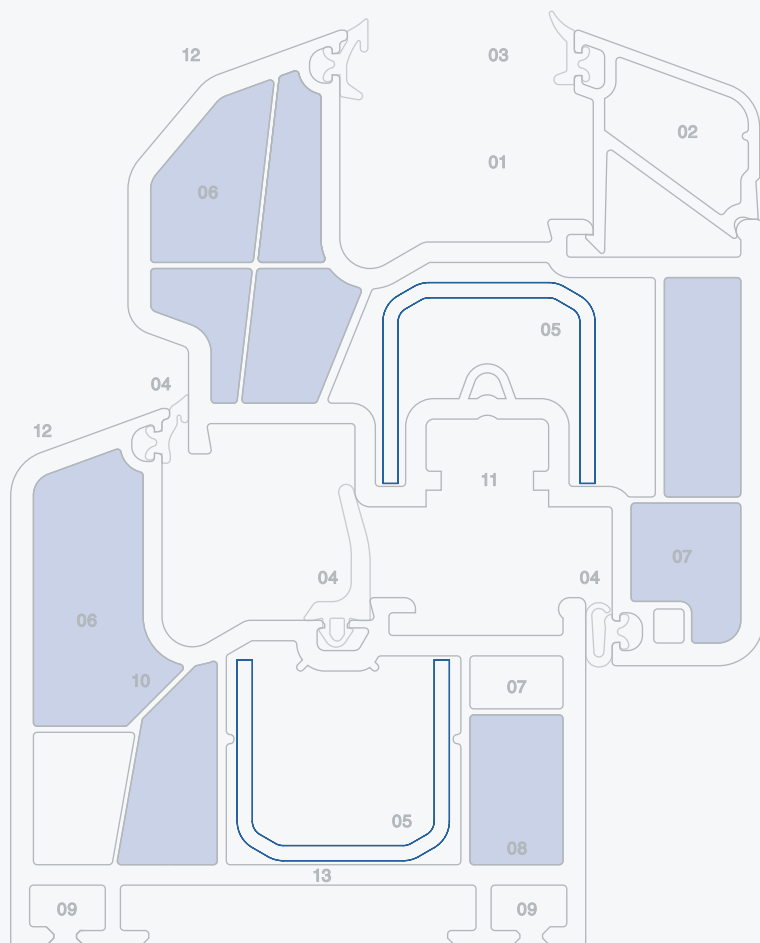
Prestige varianta s vysokou tepelnou izolací I 76.4 C4 těsnění uprostřed (MD)
